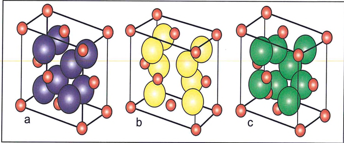
Şekil 2. 14 Zirkonyanın kristalografik formları a) monoklinik b) tetragonal c) kübik
