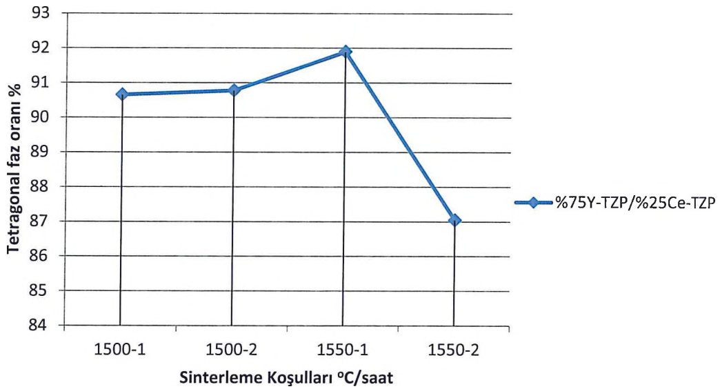
Şekil 4. 42 %75Y-TZP/%25Ce-TZP'nin tetragonal faz oranı
