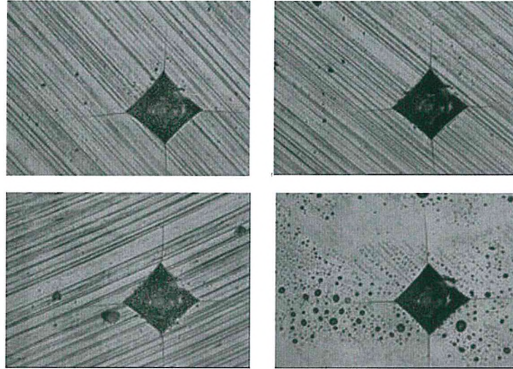
Şekil 4. 6 1500 °C 1 saat sinterlenmiş %100Y-TZP numunesi Vickers sertlik izleri
