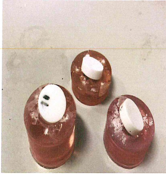
Şekil 3. 15 XRD için kalıptan çıkartılan numuneler
