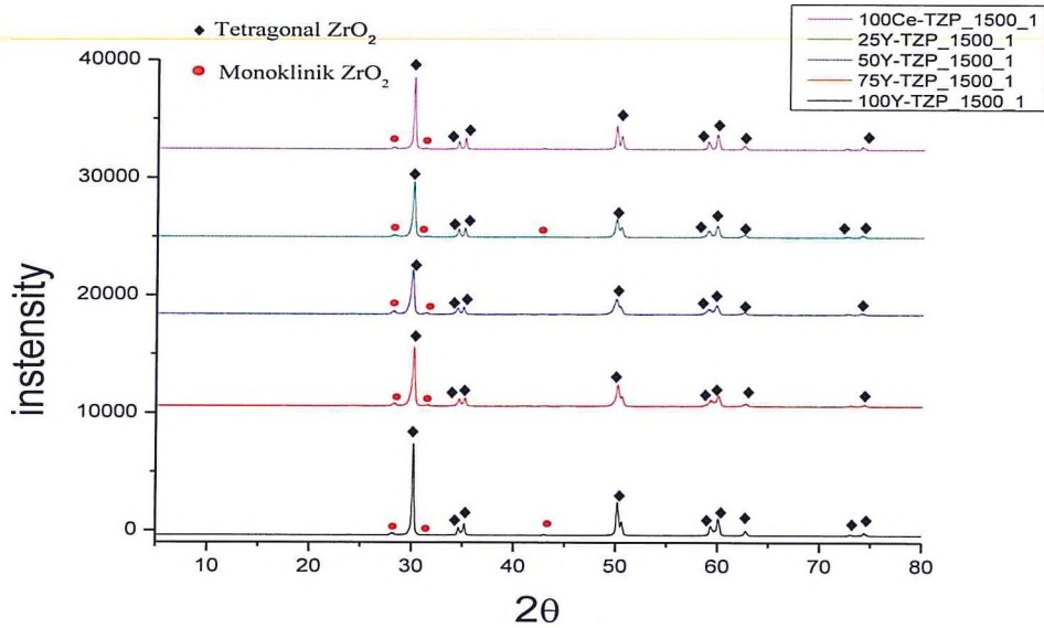
Şekil 4. 29 1500^{\circ}\text{C} - 1 Saat Sinterlenen Numunelerin XRD paternleri
