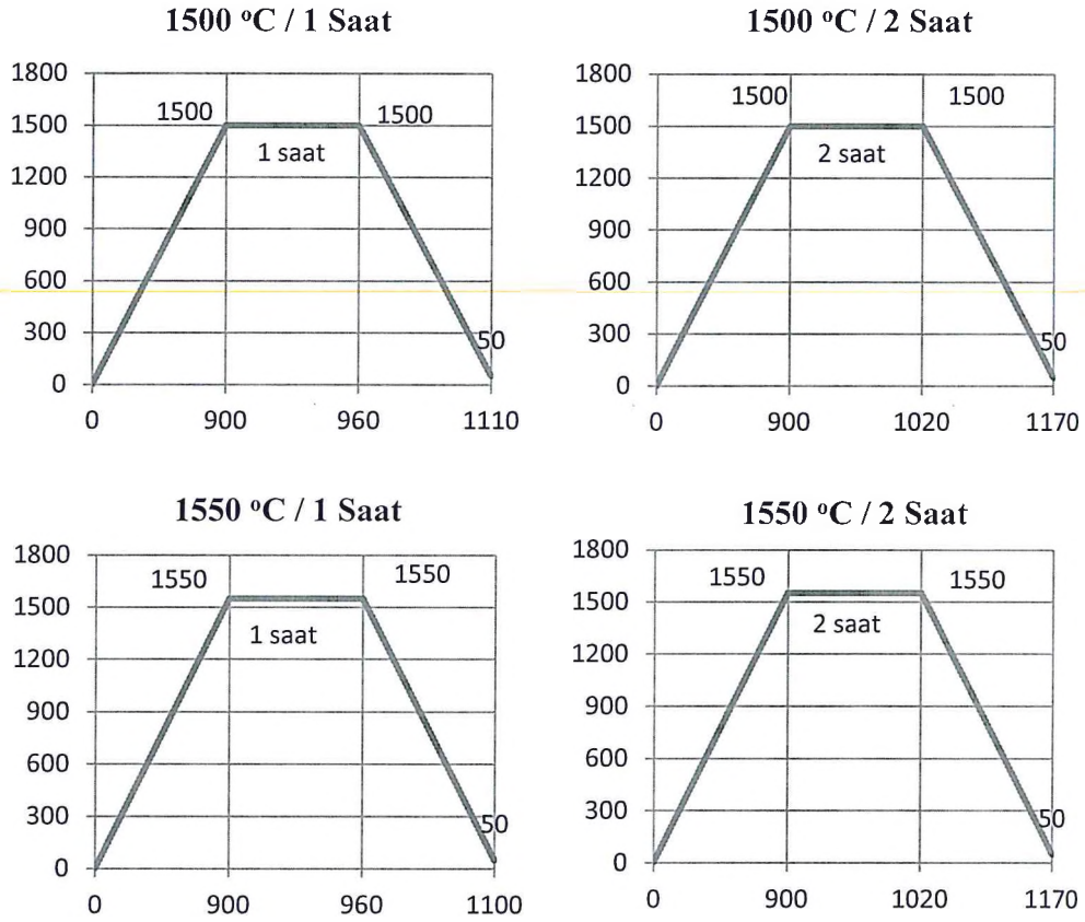
Şekil 3. 8 Sinterleme aşamaları
