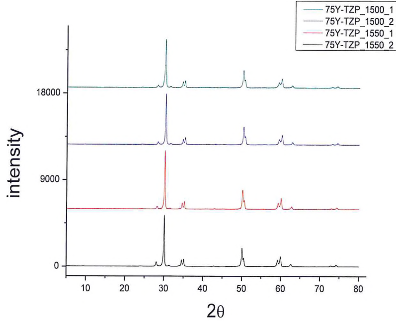
Şekil 4. 41 %75Y-TZP/%25Ce-TZP'nin XRD paternleri
