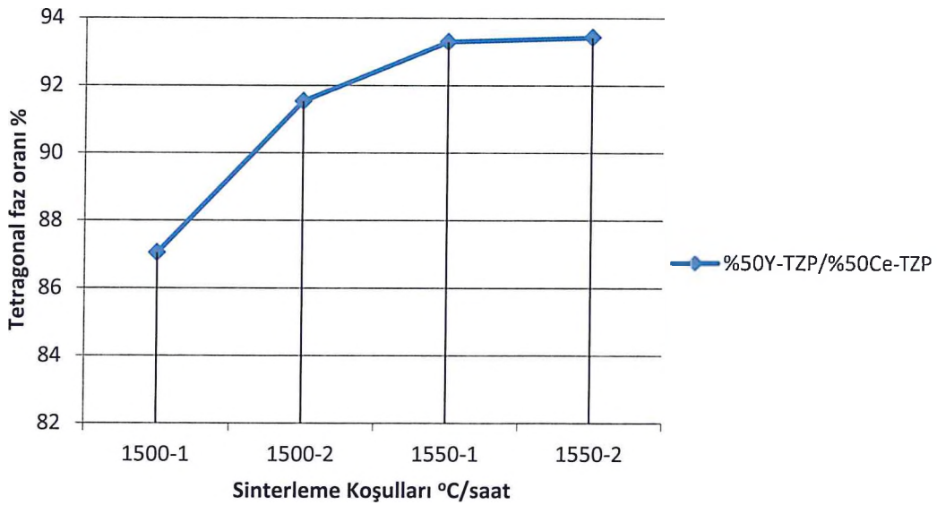
Şekil 4. 44 %50Y-TZP/%50Ce-TZP'nin tetragonal faz oranı
